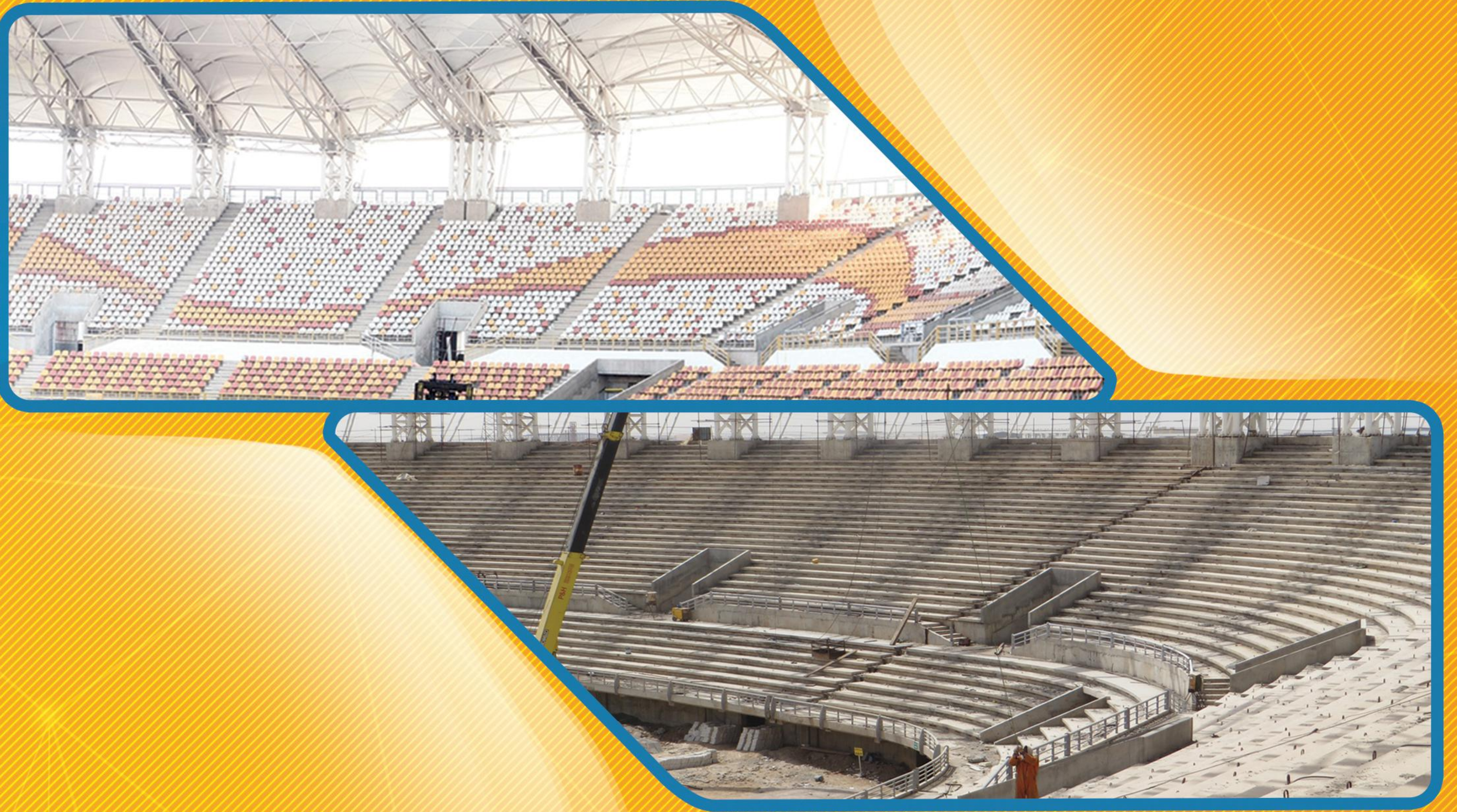
سکوهای پیش ساخته بتنی ورزشگاه فولاد خوزستان، ساخته شده توسط شرکت آبان بسیار توسعه
